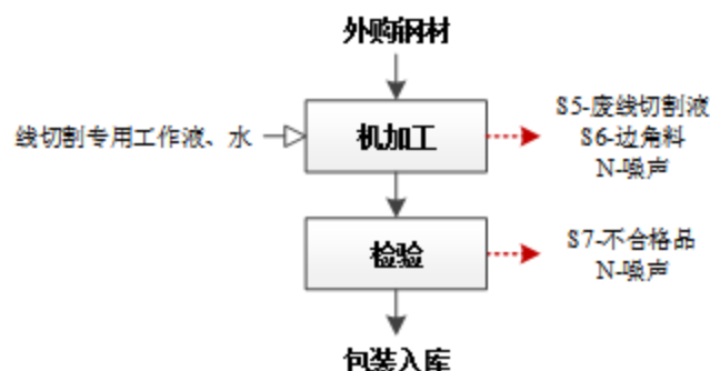
图 2-3 模具生产工艺流程图
